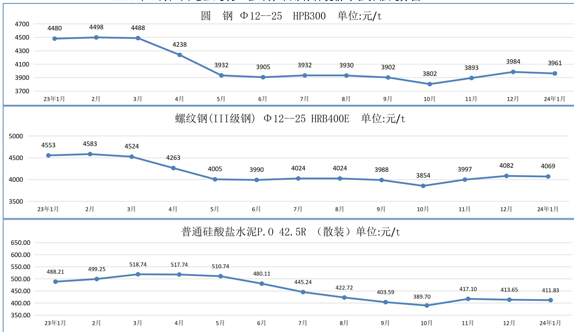
2024 年 1 月广州地区建设工程部分常用材料税前综合价格走势
